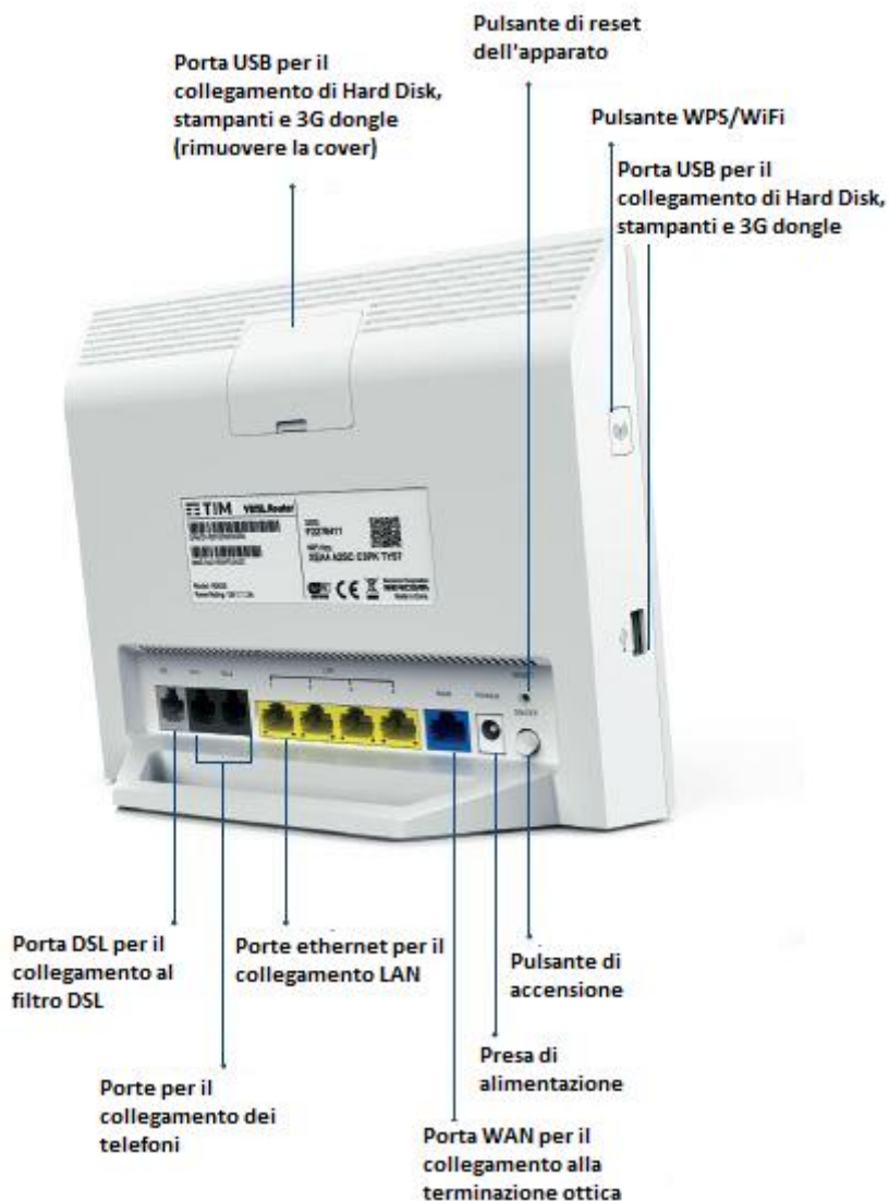
Figura 2: Pannello posteriore
